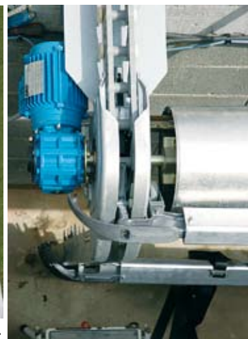
MISE EN PLACE DE LA TRANSMISSION.
